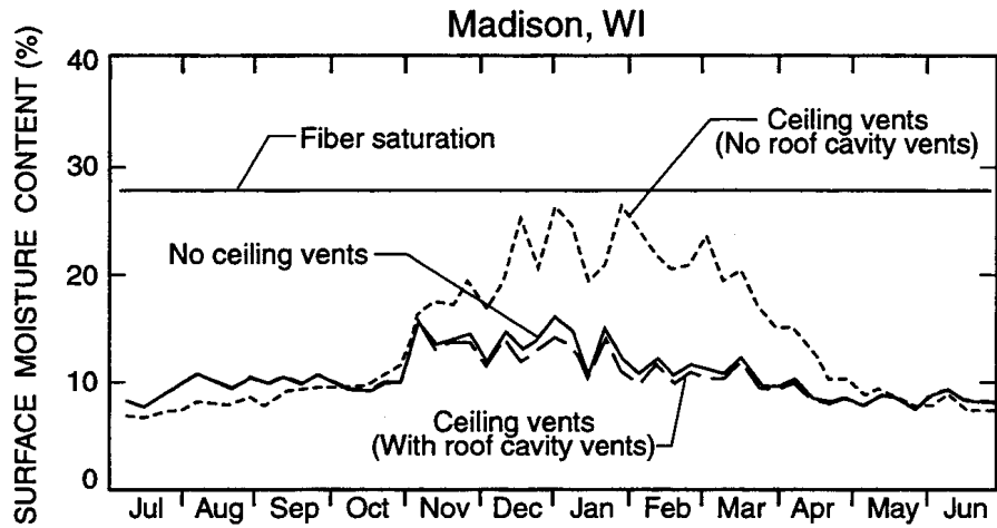
a. Surface moisture content
