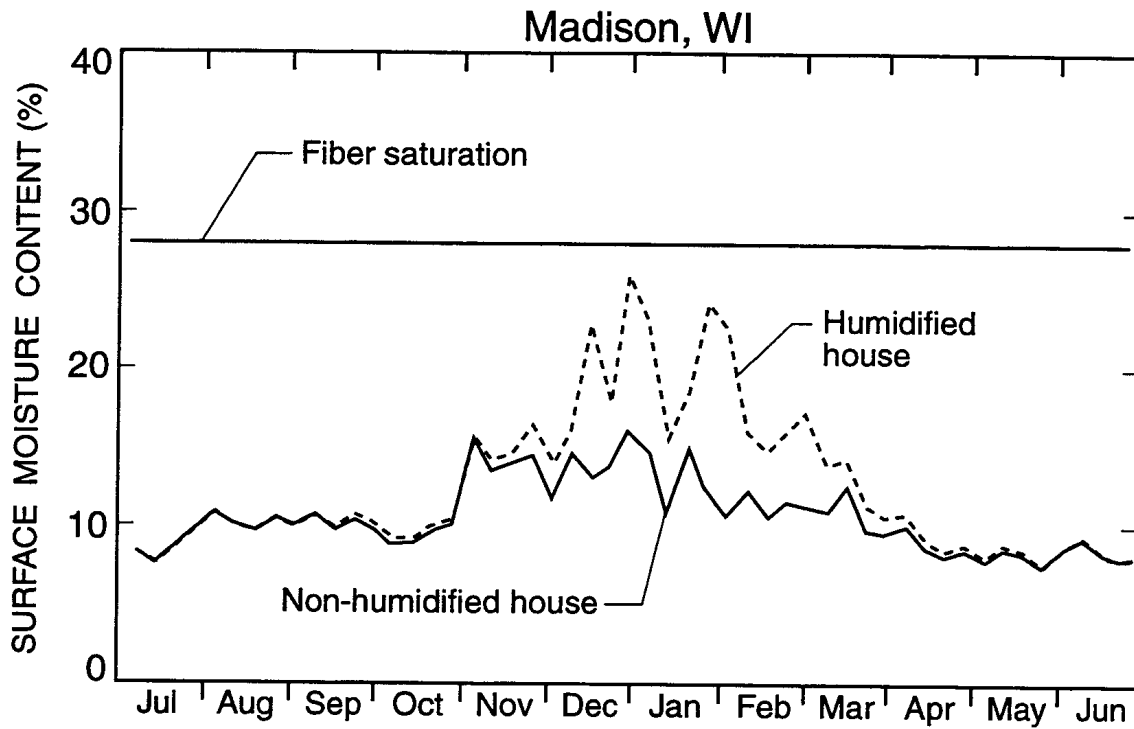
a. Surface moisture content
